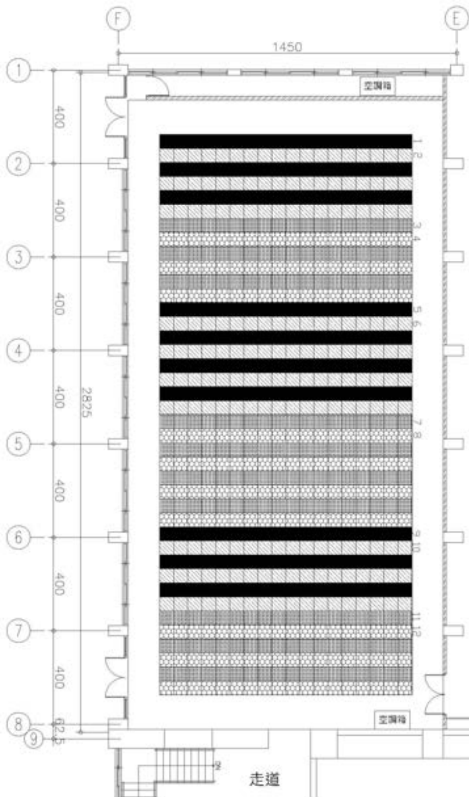
聯合餐廳展演空間一樓 LED 平板燈 平面圖
